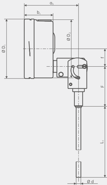
外壳旋转范围约为 < 90°
